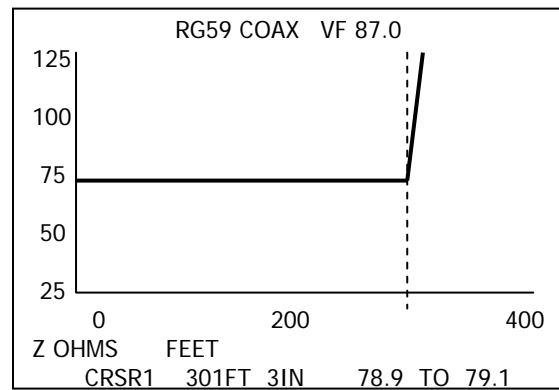
Open End – Step TDR
